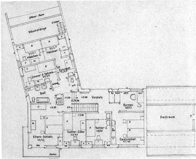
Grundrisse Maßstab 1 : 300
