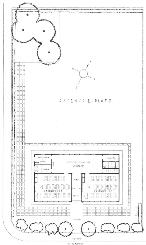
Grundriss 1:400
