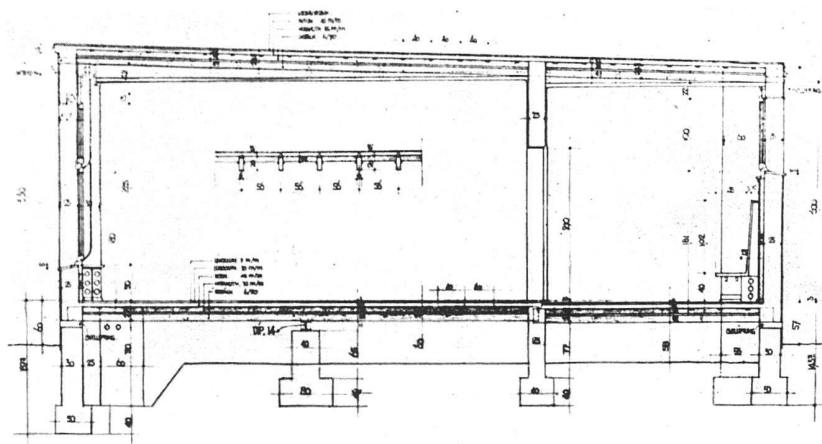
Querschnitt 1:100
