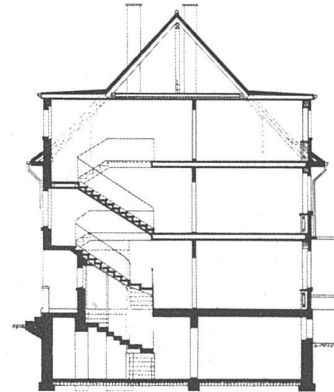
Schnitt
