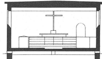
Schnitt 1 : 200
