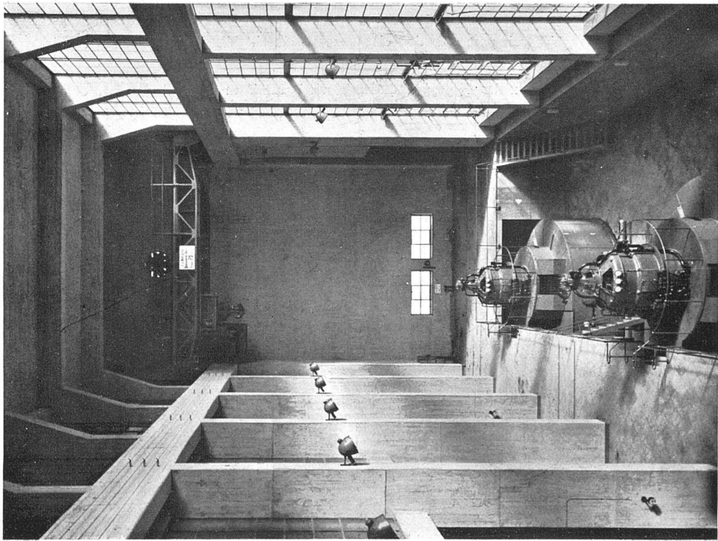
Limmatwerk Wettingen, Maschinenhaus. Architektonische Bearbeitung Gebrüder Pfister, Architekten BSA, Zürich
