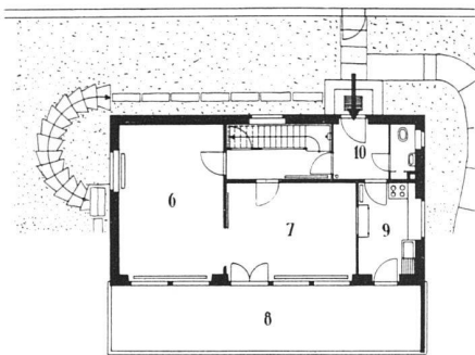
Erdgeschoss
