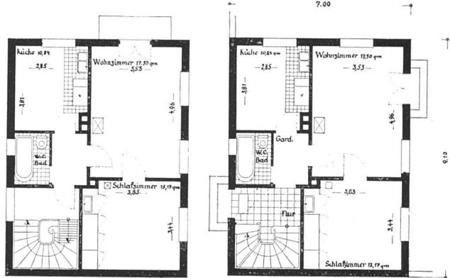
Reihenhauszeile von Arch. Emil Freymuth, Ostseite vom «Anger» gesehen, links Grundrisse 1:200
