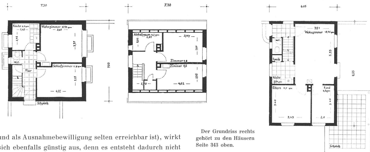
Grundrisse 1:200
