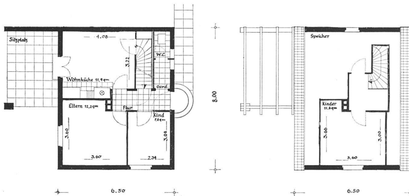
Grundrisse 1: 200
