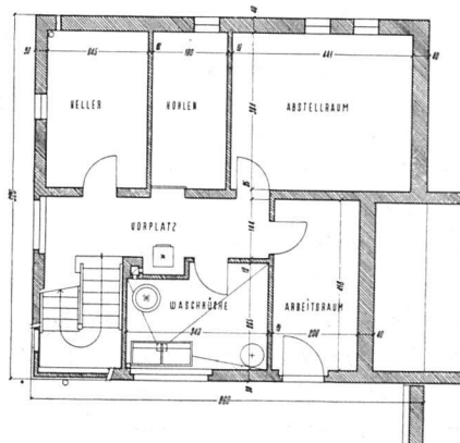
Grundrisse Kellergeschoss und Erdgeschoss 1:200
