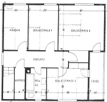
Grundriss Obergeschoss 1:200
