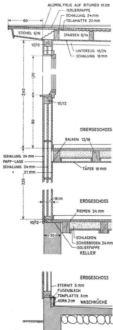
Konstruktionsdetail 1:40
