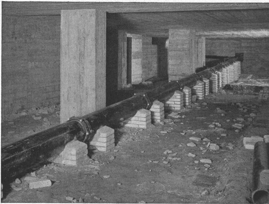
Eine der grossen Ablaufleitungen von 300 mm Ø
