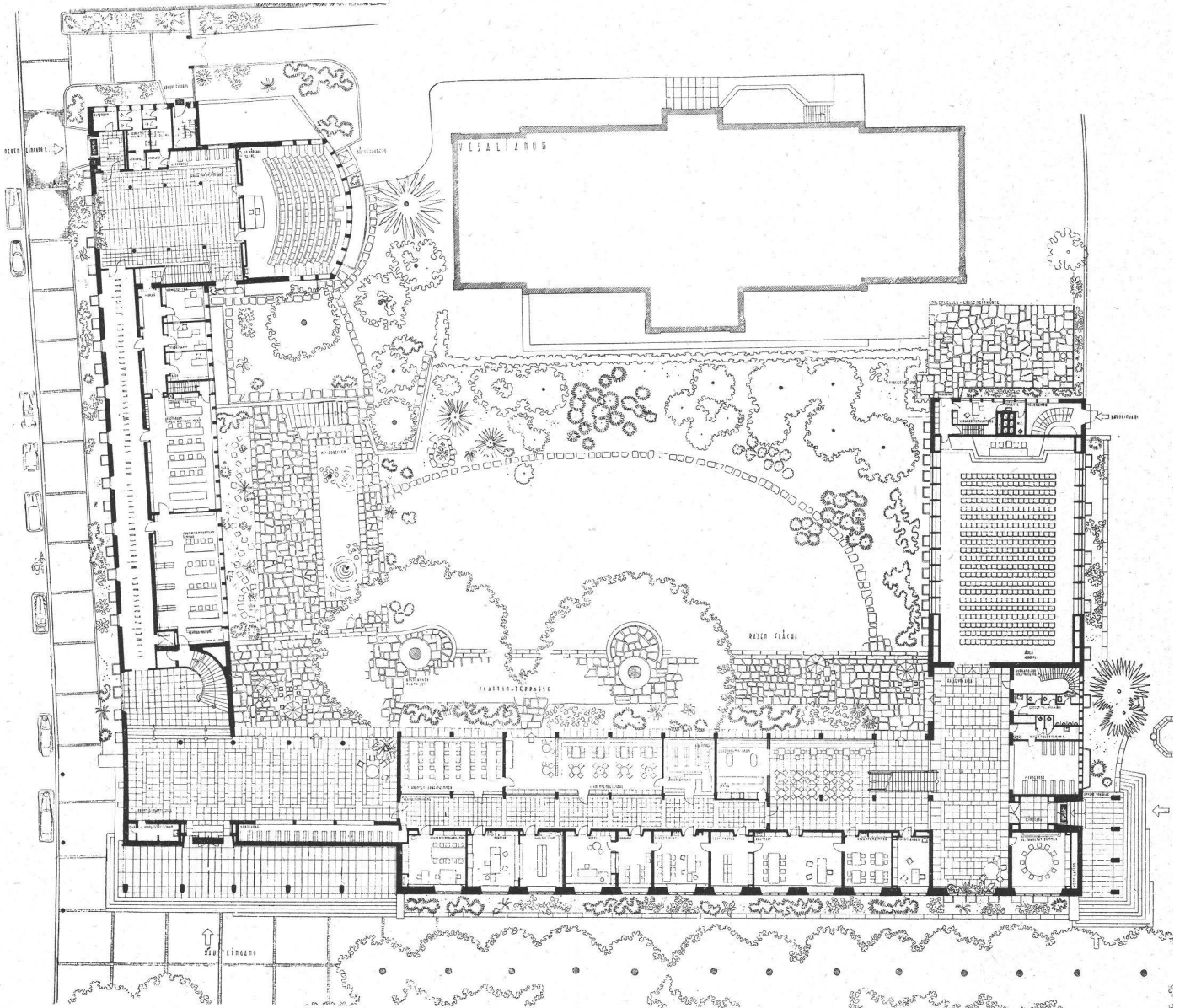
Grundriss Erdgeschoss 1 : 700 links Petersgraben, unten Petersplatz, links oben grosse Hörsäle, rechts Mitte Aula
