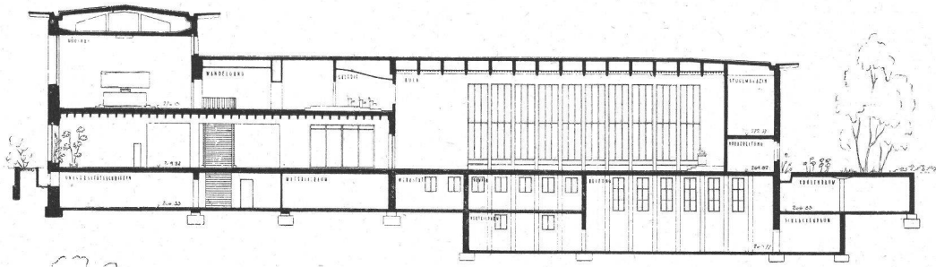
Schnitte 1 : 500 oben: Längsschnitt durch Aula, Querschnitt durch Hauptbau Petersplatz Mitte links: Querschnitt durch Hauptbau Mitte rechts: Längsschnitt durch die grosse Hörsäle, links Petersgraben
