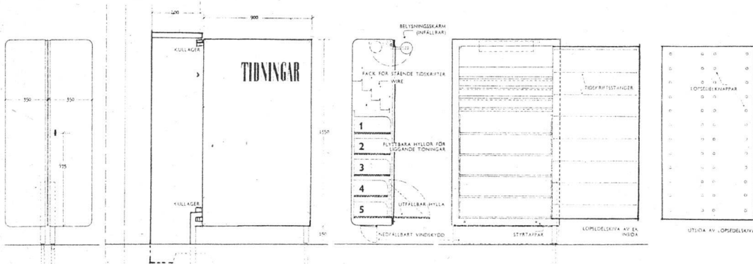
Verkaufsstand für Zeitungen (Massstab 1:40); er lässt sich wie ein Koffer öffnen; rotes lackiertes Blech, auf der Innenseite verstellbare Tablars, ausstellbare Laufzettelscheiben und elektrische Beleuchtung.
