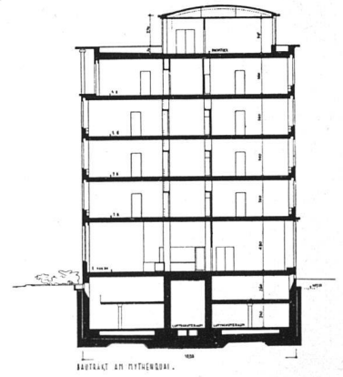
Querschnitt Bürotrakt 1:600
