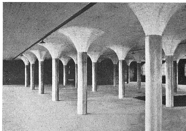
Ing. Maillart, Lagerhaus in Zürich, 1910. Erste Pilzsäulenkonstruktion in Europa
