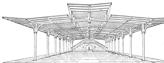
Eisenkonstruktion an der Fisch-Markthalle Hungford, London, mit Baldachin, 1835
