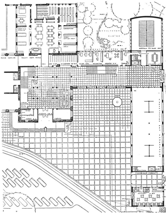
Erdgeschoß 1:1000
