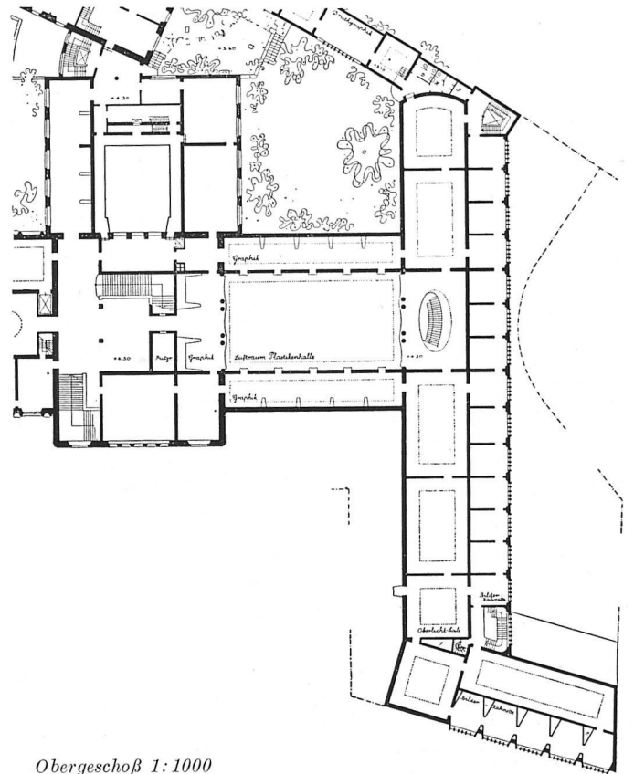
Obergeschoß 1:1000
