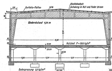
Abb. 7 Querschnitt 1:200 mit Pilsdecke für 1,5 t pro m 2 Nutzlast über Kellergeschoß und genagelte Rahmenbinder über Erdgeschoß. Spannweite ca. 17 m, Binderabstand 4,2 m
