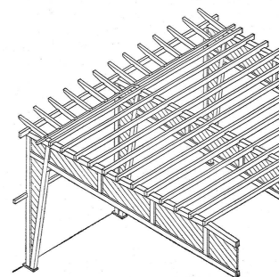
Abb. 8 Azonometrie der Holzkonstruktion mit durchlaufenden Sparren über den Rahmenbindern. Vordach mit Gegengefälle und zurückverschober Rinne
