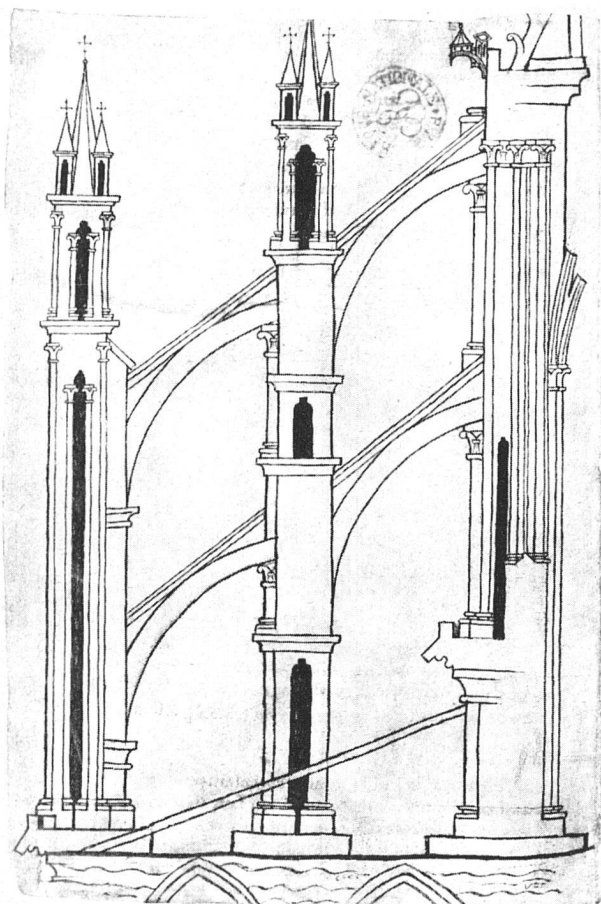
Villard de Honnecourt, Strebensystem des Reimser Chors nach unausgeführten Plane. Nach Hahnloser, Villard de Honnecourt
