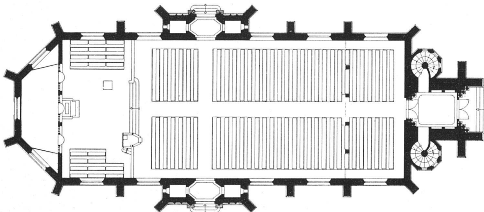
Grundriß und Schnitt 1:300 nach der Renovation
