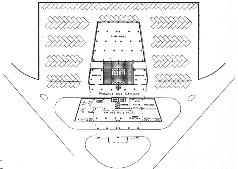
Zweites Untergeschoß 1:1700 mit Garage | Premier sous-sol, garage | First basement, garage
