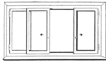
Horizontal (Fenster u. Türen) Detail 1:1, Nr. 11, 14-17
