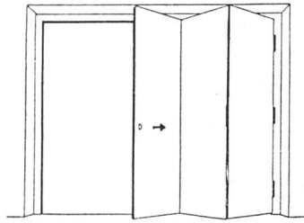
Innere Falлтüre Detail 1:1, Nr. 20
