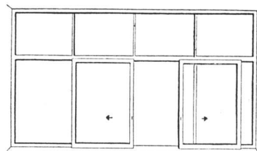
Schiebefenster Detail 1:1, Nr. 18
