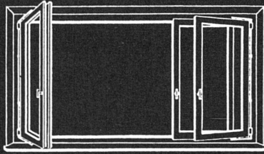
Horizontal-Drehflügel Detail 1:1, Nr. 12 und 13
