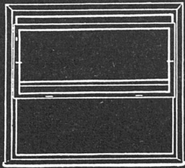
Vertikal-hochschiebbar Detail 1:1, Nr. 1-4 und 7
