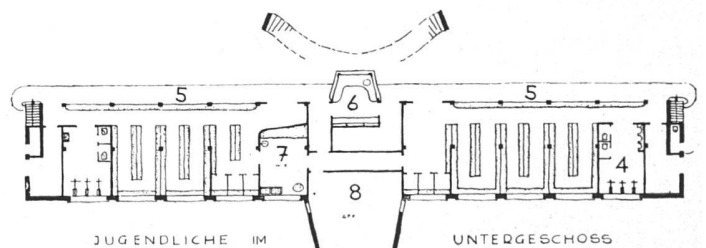
Untergeschoß für Jugendliche 1:300 | Sous-sol, vestiaires scolaires | Basement floor for children
