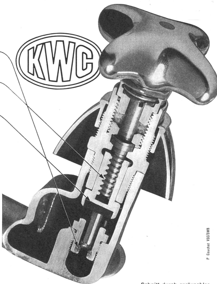
Schnitt durch geräuschlos funktionierenden Hahn
