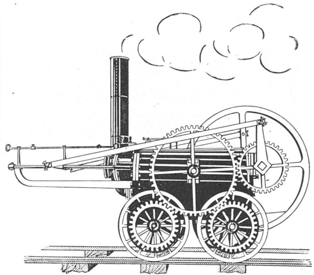
Altteste Schienenlokomotive von Trevithik, 1803
