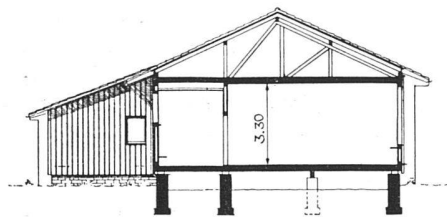
Standard-Pavillon (Ahornstraße, In der Probstei) Grundriß und Schnitt 1:300 | Pavillon standard, plan et coupe | Standard classroom wing; plan and section
