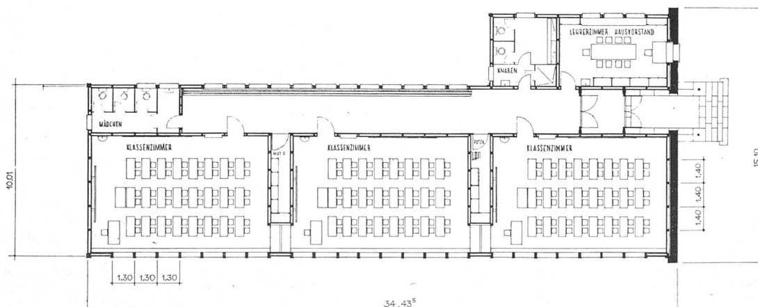
Standard-Pavillon (Ahornstraße, In der Probstei) Grundriß und Schnitt 1:300 | Pavillon standard, plan et coupe | Standard classroom wing; plan and section
