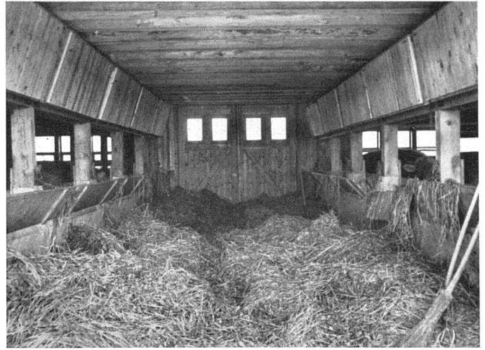
Futtertenne von der Ablad- und Dreschtenne getrennt, dadurch rationelles und sauberes Füttern | Aire de fourrage séparée de l'aire générale. Fourrage propre | Forage floor separated from threshing-floor for clean feeding
