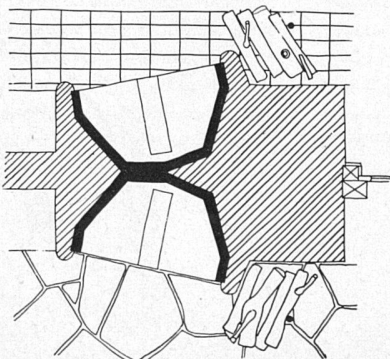
Cheminée 1:50. Feueröffnung 92 cm breit, 66 cm hoch, d.h. \frac{2}{3} der Höhe. Rauchklappe 92 cm breit, 4–10 cm tief, d.h. etwa 10% der Feueröffnung und etwa 90% des Kaminquerschnittes, der \frac{1}{8} der Feueröffnung beträgt, bei einer Kaminhöhe von 4.25 m. Die konische Rauchklappe ermöglicht die Reinigung der Rauchkammer | Cheminée | Fireplace
