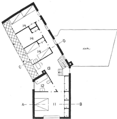
Erdgeschoß und Obergeschoß 1:300 | Rez-de-chaussée et étage | Ground-floor and upper floor
