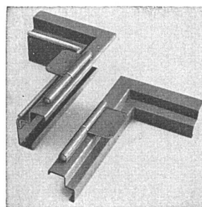
norm Türzargen
