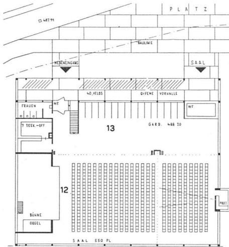
Erdgeschoss 1:600
