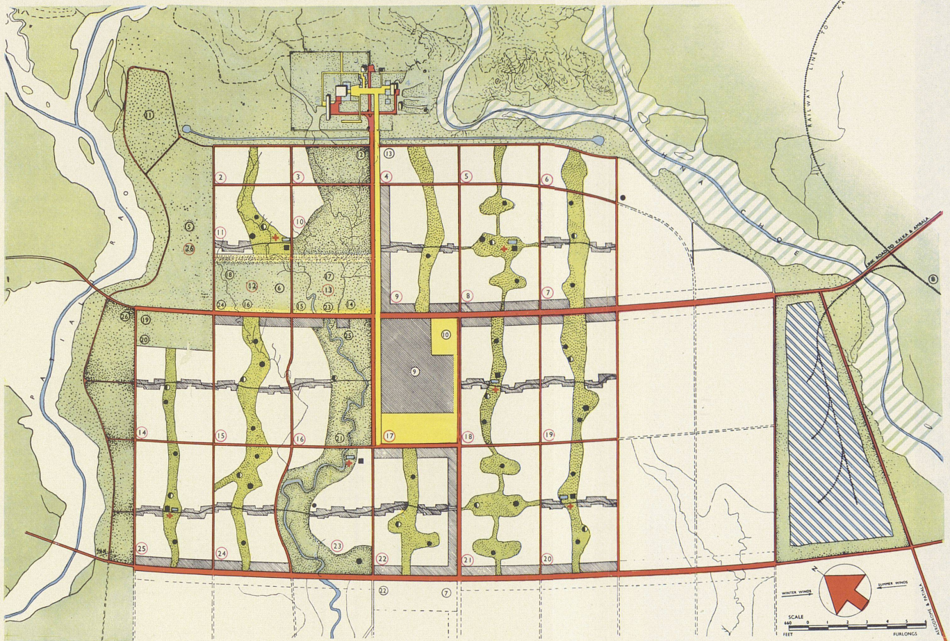
Chandigarh; Stadtplan der ersten Baustappe für 150 000 Einwohner, ca. 1:37 000 Chandigarh; plan de la ville, première étape pour 150 000 habitants Chandigarh; town-plan of the first stage for 150 000 people
