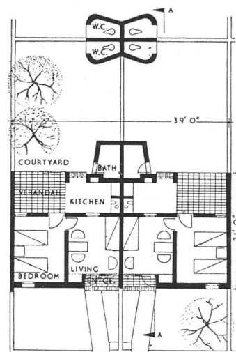
Haus-Typ 13 D 1:300 / Plan / Groundfloor
