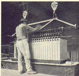
Fabrikation Alba-Platten
