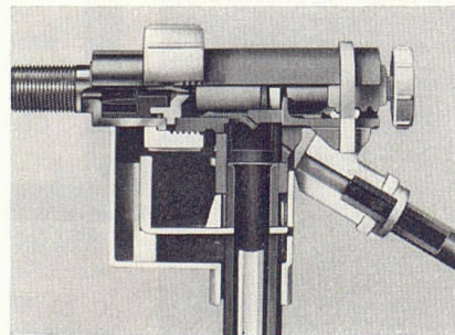
Neues GEBERIT-Schwimmventil Modell 1970.
