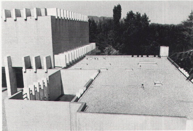
Kirchliches Zentrum Glaubten, Zürich Hescoplan T Dachhaut
