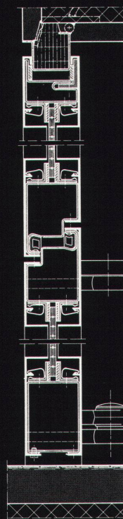
Vertikalschnitt
