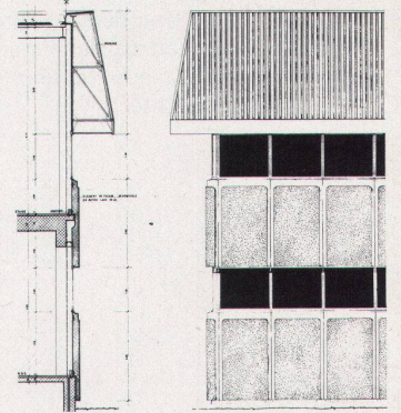
Detail der Fassade Section de détail de la façade Detail section of curtain-wall façade
