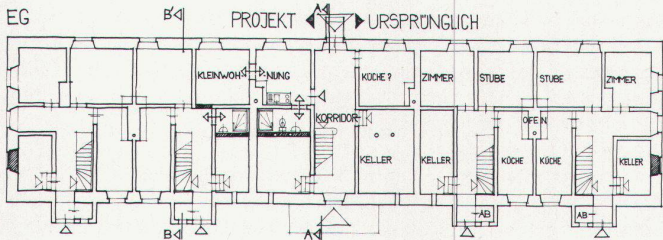
Grundriss Erdgeschoss
