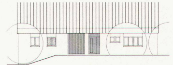
Nordwestansicht Wohnhaus
