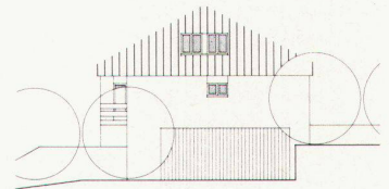
Nordostansicht Wohnhaus
