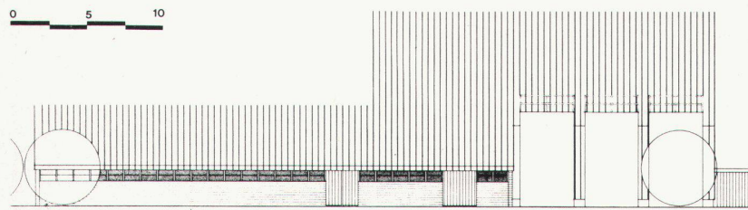
Südostansicht Scheune
