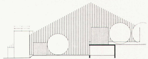
Nordostansicht Scheune
