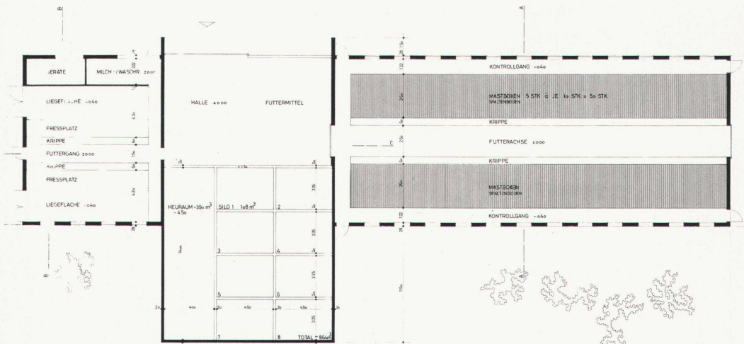
Grundriss Ökonomiegebäude
