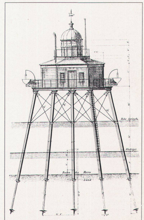
8 Phare de Belfast, 1844, d'Alexander Mitchell. Illustr.: Allgem. Bauzeitung, 15e année 1850, feuille 321
