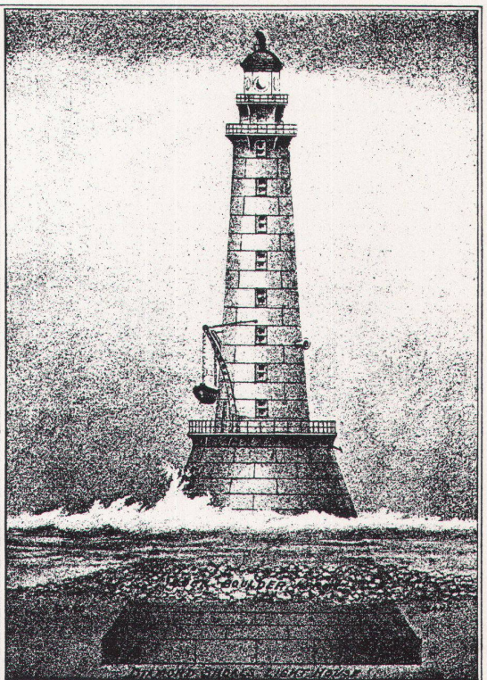
11 Der Leuchtturm am Cap Hatteras, Nord-Carolina, 1903 mit schwimmendem Fundierungskörper auf sandigem Meeresboden erbaut. Bildquelle: Prometheus, 17. Jg., 1906, S. 731
