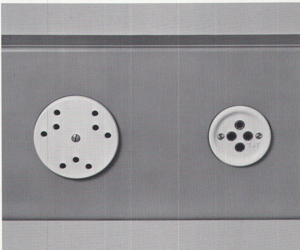
Starkstrom- und T+T-Steckdose in Installationskanal eingebaut
