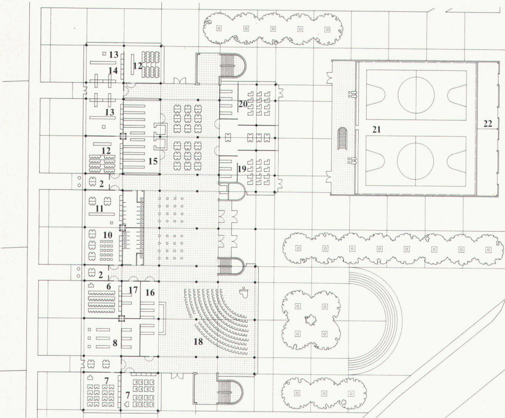
Grundriss Erdgeschoss
