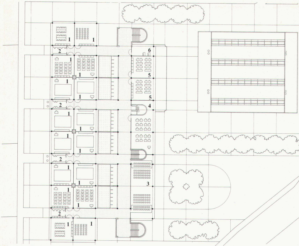
Grundriss Obergeschoss
