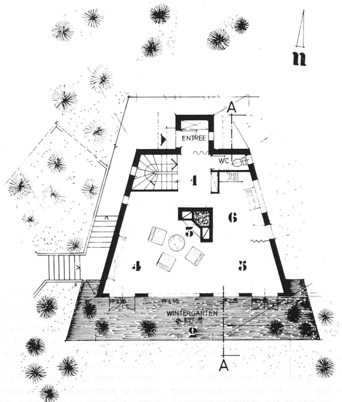
35 Grundriss Erdgeschoss/plan rez-de-chaussée. 1. Thermische Pufferzonen Nord/zones de tampon nord; 2. Thermische Pufferzonen Süd/zones de tampon sud; 3. Zentralkamine/cheminées centrales; 4. Wohnraum/séjour; 5. Essraum/manger; 6. Küche/cuisine.
