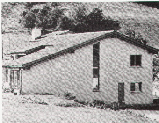
- Doppel-Einfamilienhaus, Meierskappel. 1980. Aussenisolation.
