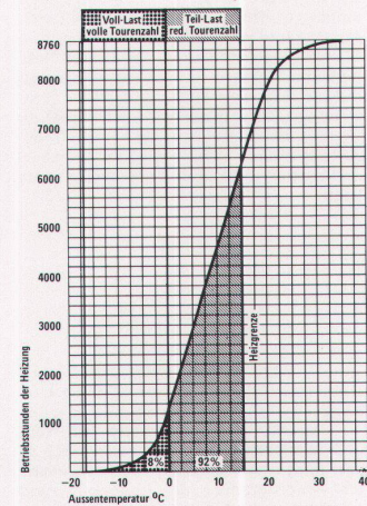
Vorteile eines 2tourigen Kompressormotors
