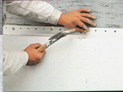
Setzen des Schlagübels.
