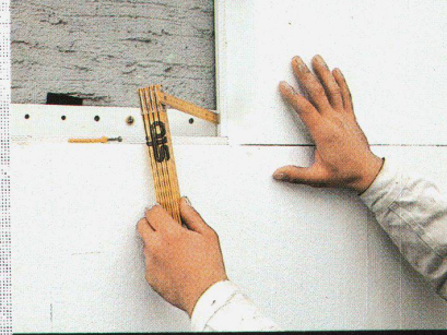
Einsetzen der Fassaden-Dämmplatten.
