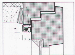
Fensteranierung HEBGO 121/526
