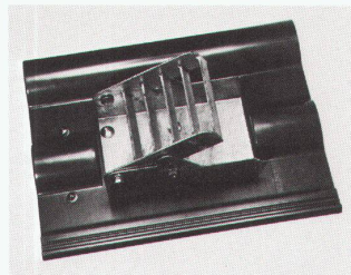
Standon-Dachflächen-Steigtritt mit abratsicherer Trittplatte, die auf Dachneigungen zwischen 20° und 50° eingestellt werden kann.
