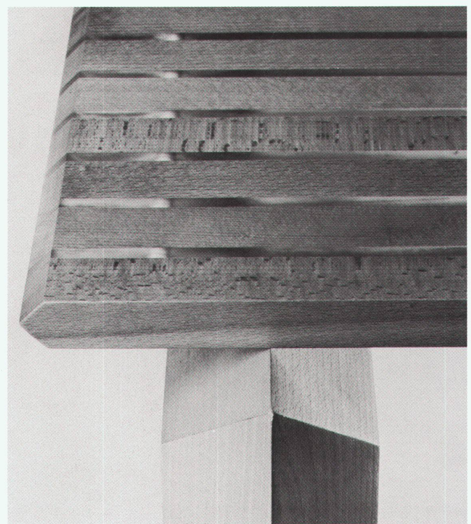
7. 8. Rang: «Pliss», Kat. C. Lukas Meier. Tisch mit einer Platte aus untereinander verleimten Buchenholz- und Plexiglasstreifen / 4ème prix: «Pliss», cat. C. Lukas Meier. Table à dessus constitué de bandes de hêtre et de plexiglas collées les unes aux autres.
