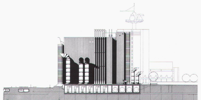
11 Südansicht / Vue sud / View from the south
