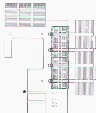
11 12 Erdgeschoss und Obergeschoss (Abstimmungsprojekt) / Rez-de-chaussée et étage (projet du jugement) / Ground floor and upper floor (voting project)
