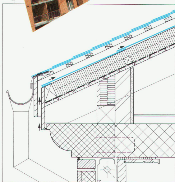
Dachaufbau von unten nach oben: Dachschiefer, Dampfsperre, Wärmedämmung, GEA-Unterdach, Konterlattung, Lattung, Dachschiefer 60/40 cm in Doppeldeckung, Farbe Pastellblau.
